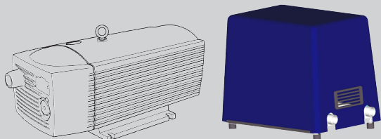
Vakuumpump 685950, för täta laster Tillval: Ljuddämpande huv 666730
