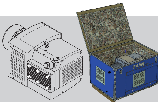
Vakuumpump 685960, för otäta laster Tillval: Ljuddämpande låda 666720
